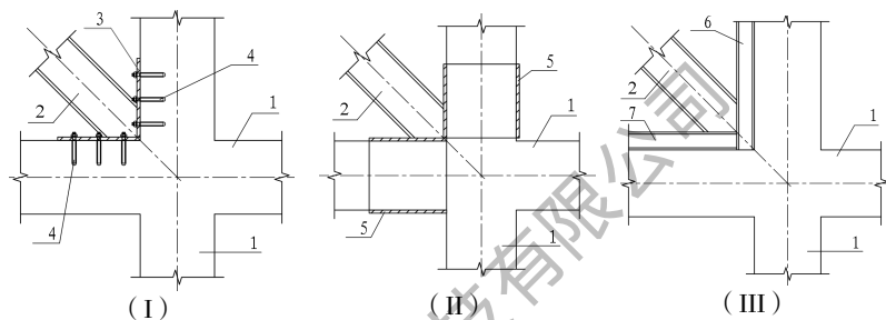
图 A.0.2-1 钢支撑与现浇混凝土框架节点域连接构造
